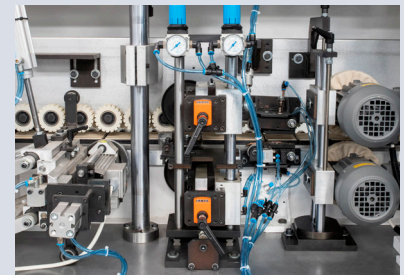
Radyüs Kazıma Ünitesi Radius Scrapper Unit
