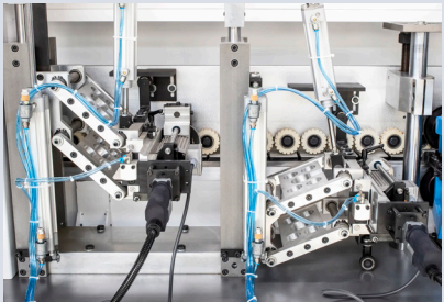
Servo Kontrollü Köşe Yuvarlama Ünitesi Rounder Unit With Servo Control
