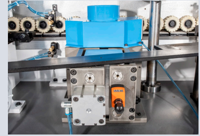
Ön Freze Ünitesi Pre Milling Unit
