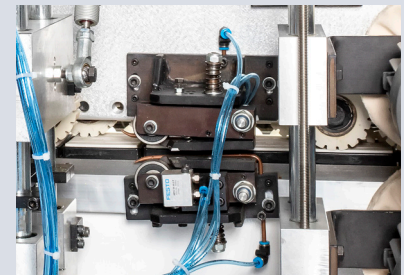
Tutkal Kazıma Ünitesi Glue Joint Scrapper
