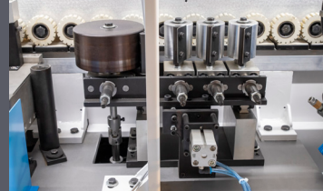
Otomatik Ayarlı Baskı Merdaneleri Autoset Pressure Rollers
