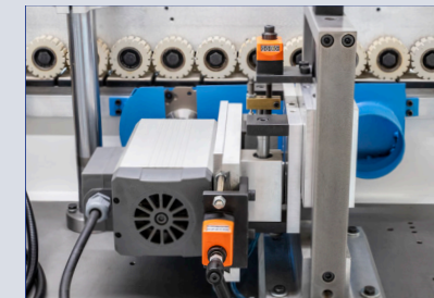
Jumpingli Kanal Testere Ünitesi Jumping Grooving Saw Unit
