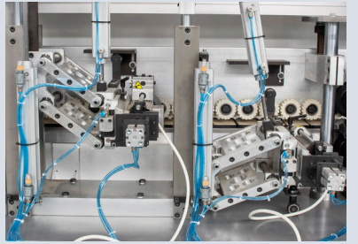
Otomatik Ayarlı Köşe Yuvarlama Ünitesi Autose Rounder Unit
