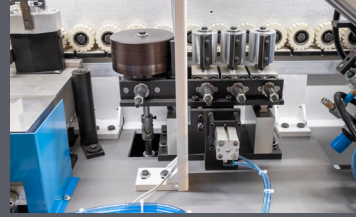
Otomatik Ayarlı Baskı Merdaneleri Autose Pressure Rollers
