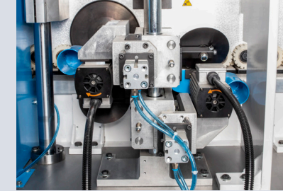
Otomatik Ayarlı Freze Ünitesi Autoset Milling Unit
