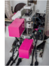
Ön Freze Ünitesi (0-3 mm) Pre Milling Unit (0-3 mm)
