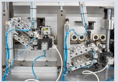
Otomatik Ayarlı Köşe Yuvarlama Ünitesi Autoset Rounder Unit
