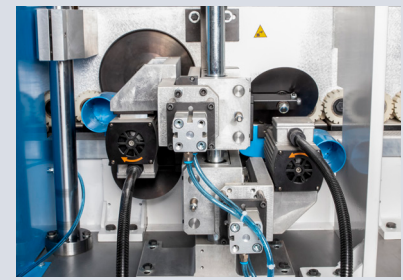
Otomatik Ayarlı Freze Ünitesi Autoset Milling Unit
