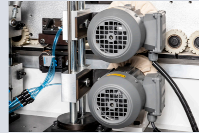
Polisaj Ünitesi Buffing Unit
