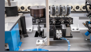
Otomatik Ayarlı Baskı Merdaneleri Autose Pressure Rollers
