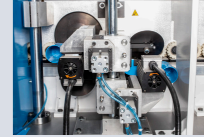
Otomatik Ayarlı Freze Ünitesi Autose Milling Unit
